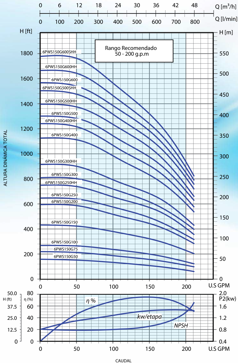
6PWS150G Curvas de Rendimiento
