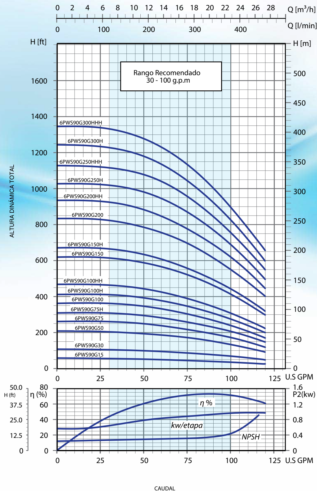
Curvas de Rendimiento - 6PWS90G
