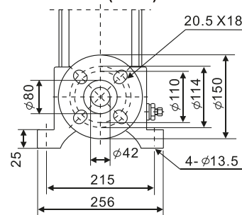
FGJ(DIN-ANSI-JIS) PN25(DN40)
